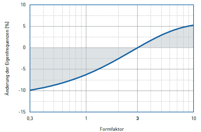
Eigenfrequenz
